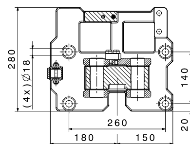
Schnitt A-A section
